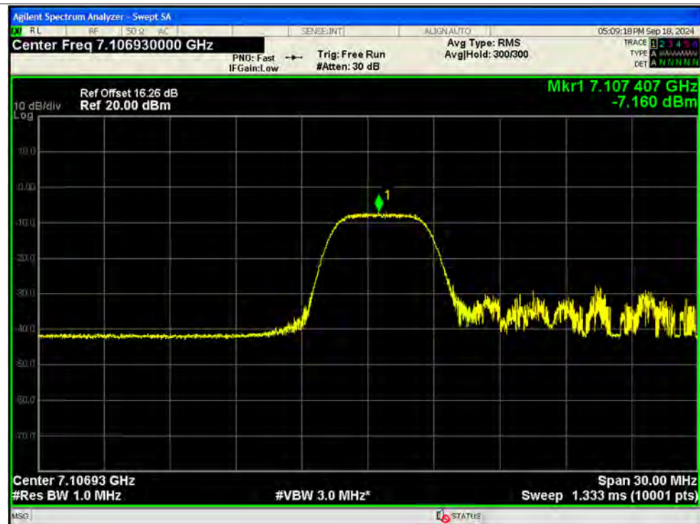
PSD NVNT be20 52@37 7115MHz Ant13 MIMO
