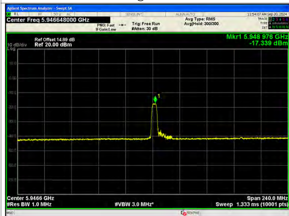
PSD NVNT be160 52@74 6025MHz Ant12 MIMO
