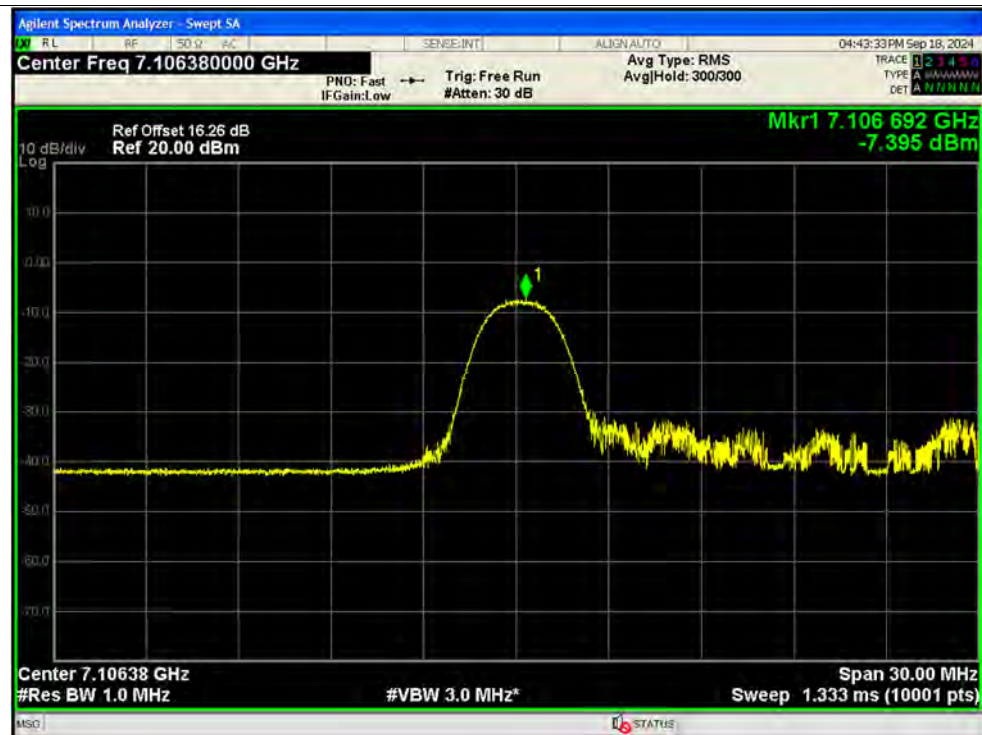
PSD NVNT be20 26@0 7115MHz Ant13 MIMO
