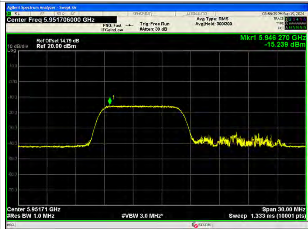
PSD NVNT ax20 106@53 5955MHz Ant13 MIMO
