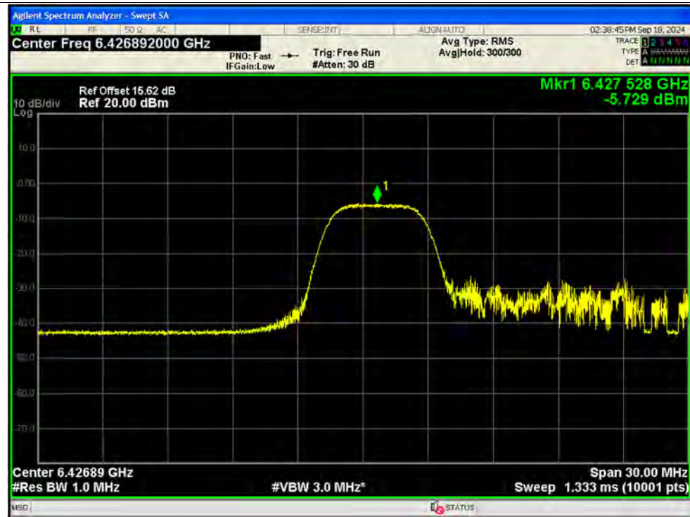
PSD NVNT ax20 52@37 6435MHz Ant13 MIMO
