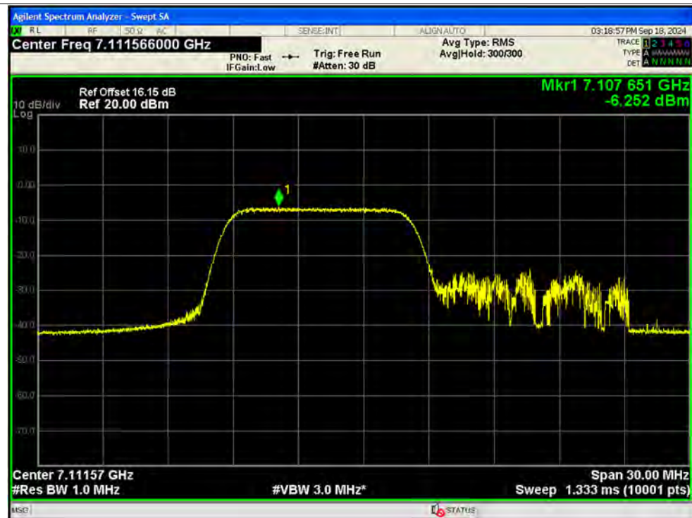
PSD NVNT ax20 106@53 7115MHz Ant12 SISO
