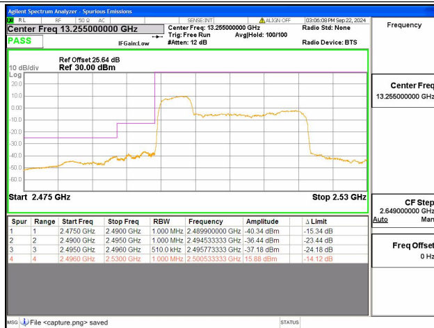
41C / 5+20MHz / Low CH / QPSK / 25#0-100#0
