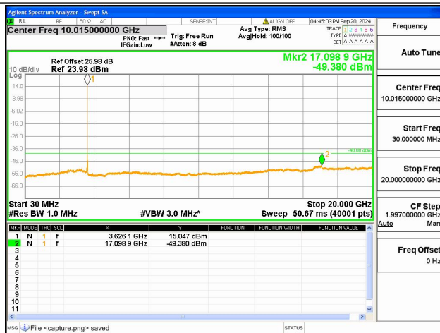
48C-30M-20G / 20+15MHz / QPSK / Mid CH / 1@99-1@0
