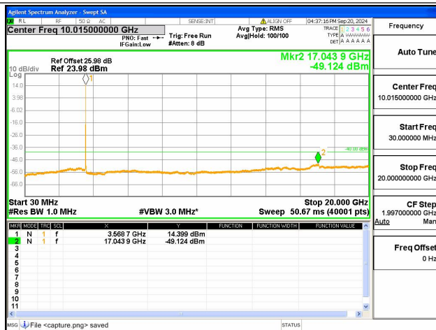
48C-30M-20G / 20+20MHz / QPSK / Low CH / 1@99-1@0
