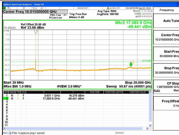
48C-30M-20G / 20+5MHz / QPSK / Mid CH / 1@99-1@0
