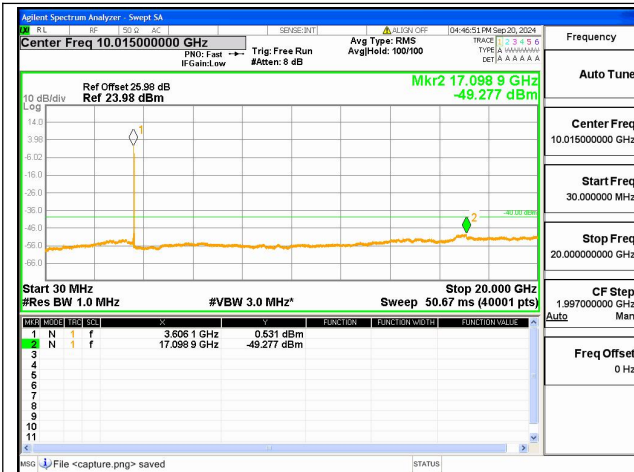
48C-30M-20G / 20+20MHz / QPSK / Mid CH / 1@0-1@99
