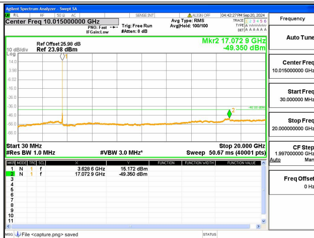
48C-30M-20G / 20+10MHz / QPSK / Mid CH / 1@99-1@0
