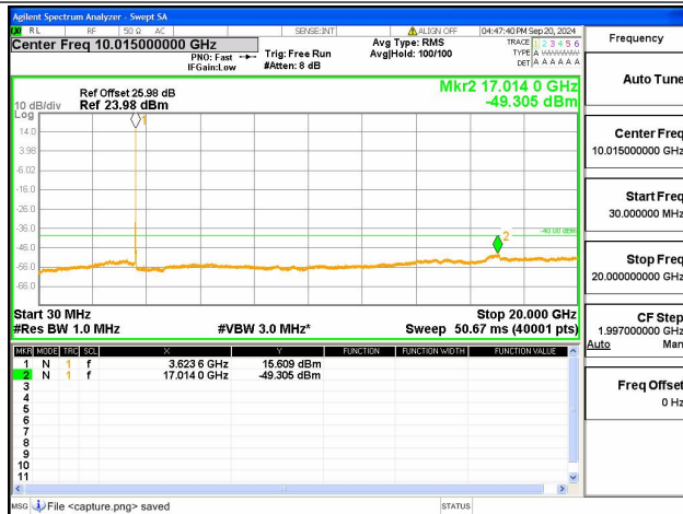
48C-30M-20G / 20+20MHz / QPSK / Mid CH / 1@99-1@0
