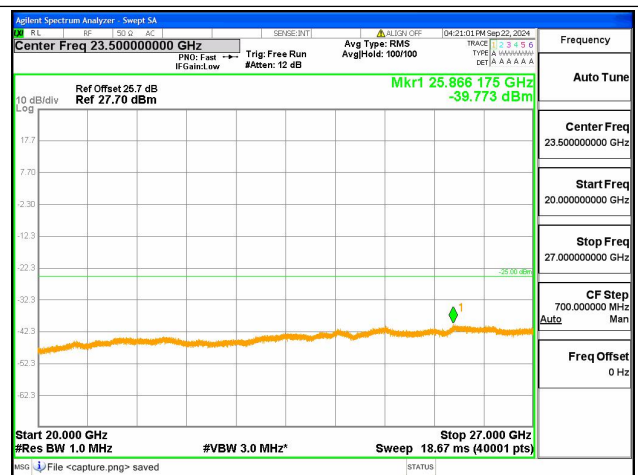
41C-20G-27G / 20+20MHz / QPSK / Mid CH / 1@0-1@99
