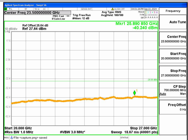
41C-20G-27G / 20+10MHz / QPSK / Low CH / 1@0-1@49
