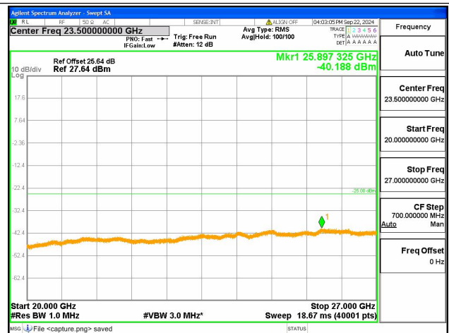
41C-20G-27G / 20+10MHz / QPSK / Low CH / 100@0-50@0
