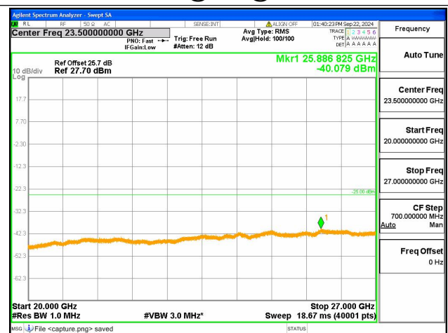
41C-20G-27G / 10+20MHz / QPSK / Mid CH / 50@0-100@0
