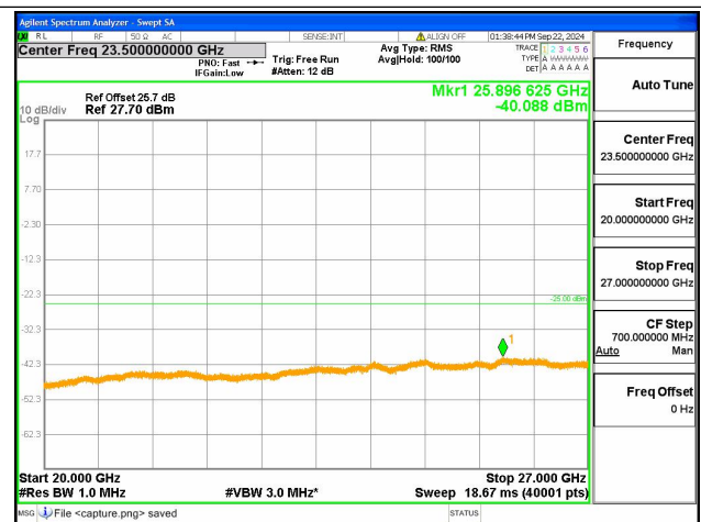
41C-20G-27G / 10+20MHz / QPSK / Mid CH / 1@0-1@99
