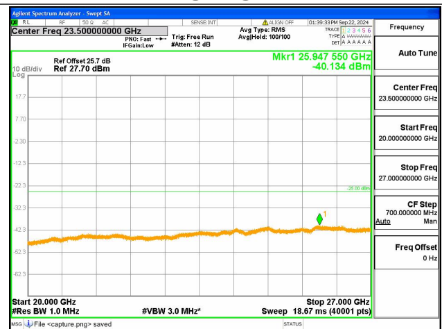
41C-20G-27G / 10+20MHz / QPSK / Mid CH / 1@49-1@0
