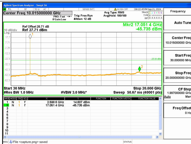
38C-30M-20G / 20+20MHz / QPSK / High CH / 1@99-1@0
