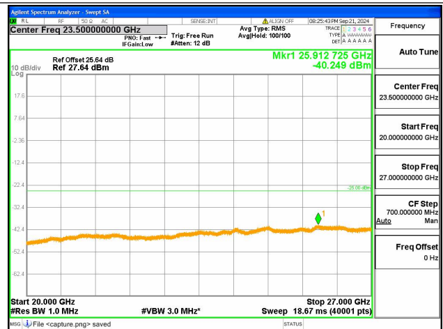
41C-20G-27G / 5+20MHz / QPSK / Low CH / 1@24-1@0
