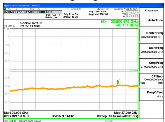
38C-20G-27G / 20+20MHz / QPSK / High CH / 100@0-100@0
