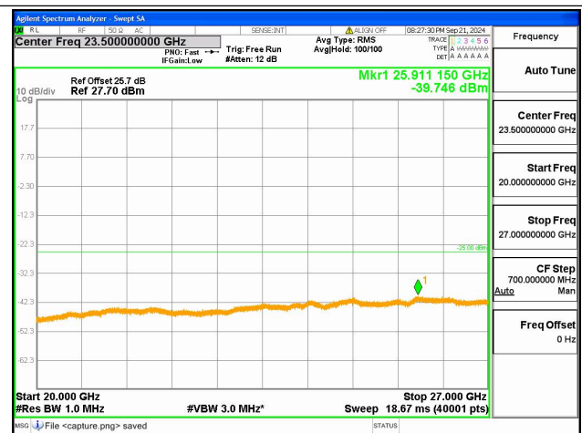
41C-20G-27G / 5+20MHz / QPSK / Mid CH / 1@0-1@99
