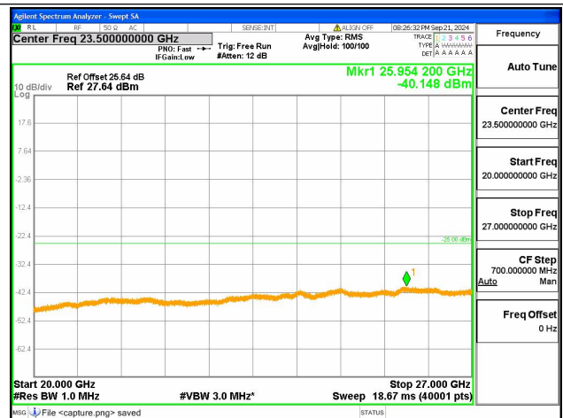
41C-20G-27G / 5+20MHz / QPSK / Low CH / 25@0-100@0
