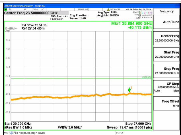
41C-20G-27G / 5+20MHz / QPSK / Low CH / 1@0-1@99
