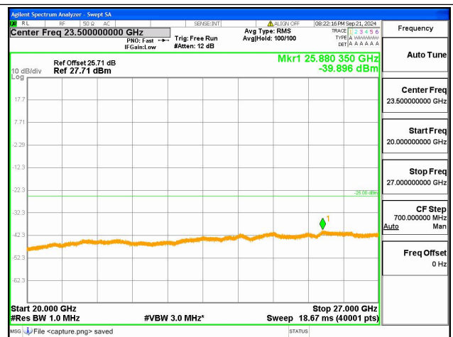
38C-20G-27G / 20+20MHz / QPSK / High CH / 1@0-1@99
