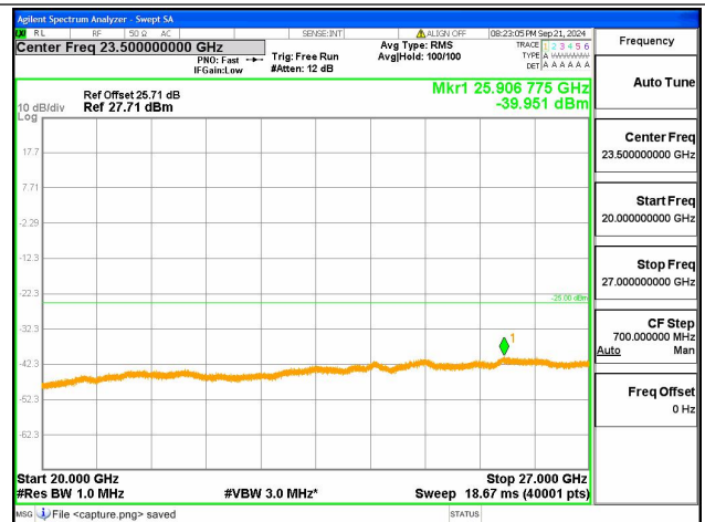
38C-20G-27G / 20+20MHz / QPSK / High CH / 1@99-1@0
