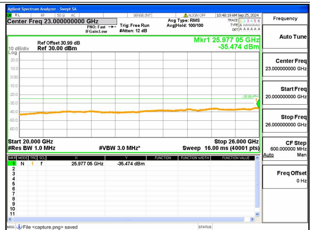
7A-12A-20G-26G / 20+10MHz / QPSK / Mid+High CH / 100@0-50@0
