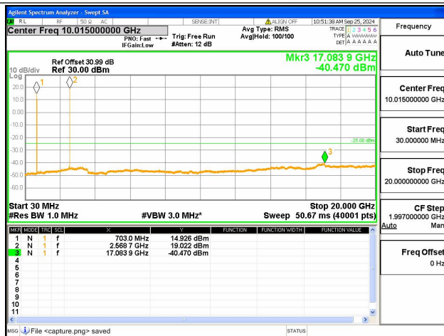
7A-12A-30M-20G / 20+10MHz / QPSK / High+Mid CH / 1@99-1@0
