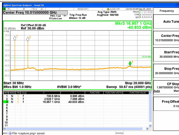
7A-12A-30M-20G / 20+10MHz / QPSK / Mid+Low CH / 100@0-50@0
