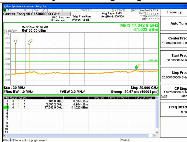
7A-12A-30M-20G / 20+10MHz / QPSK / High+Mid CH / 100@0-50@0
