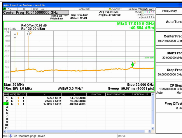
7A-12A-30M-20G / 20+10MHz / QPSK / High+Low CH / 1@99-1@0
