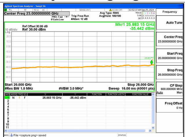
7A-12A-20G-26G / 20+10MHz / QPSK / High+Mid CH / 100@0-50@0
