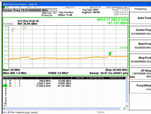
7A-12A-30M-20G / 20+10MHz / QPSK / Mid+High CH / 1@99-1@0
