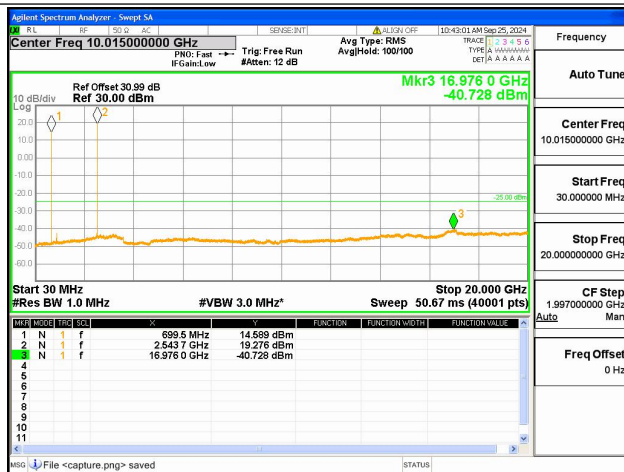
7A-12A-30M-20G / 20+10MHz / QPSK / Mid+Low CH / 1@99-1@0
