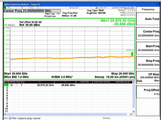
7A-12A-20G-26G / 20+10MHz / QPSK / Mid+Mid CH / 1@99-1@0
