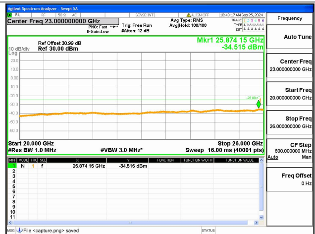
7A-12A-20G-26G / 20+10MHz / QPSK / Mid+Low CH / 1@99-1@0
