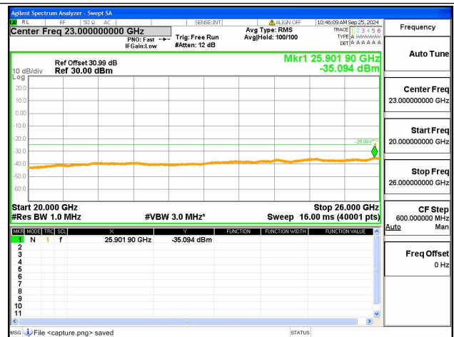
7A-12A-20G-26G / 20+10MHz / QPSK / Mid+Mid CH / 100@0-50@0
