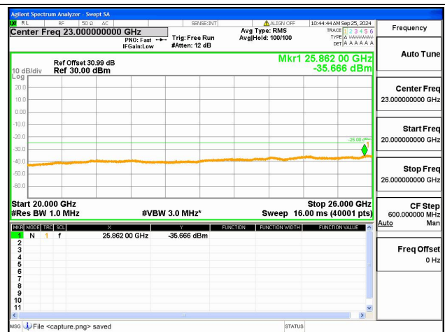
7A-12A-20G-26G / 20+10MHz / QPSK / Mid+Mid CH / 1@0-1@49
