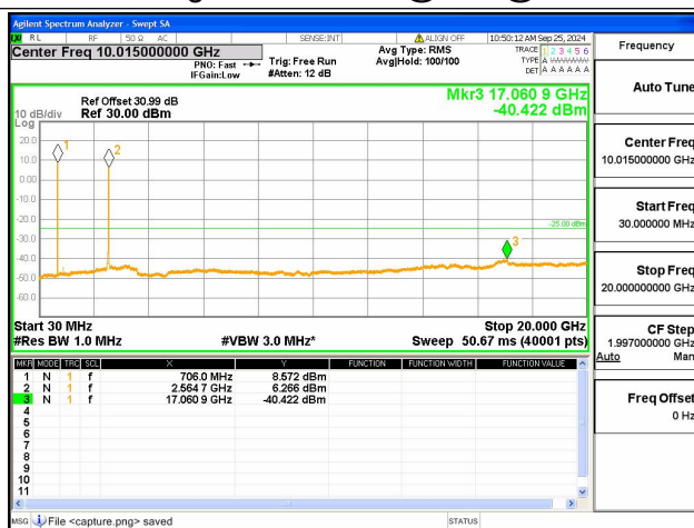
7A-12A-30M-20G / 20+10MHz / QPSK / High+Low CH / 100@0-50@0
