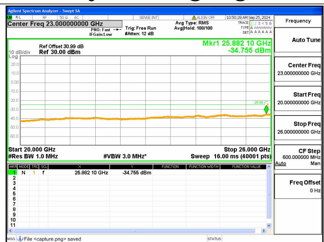
7A-12A-20G-26G / 20+10MHz / QPSK / High+Low CH / 100@0-50@0
