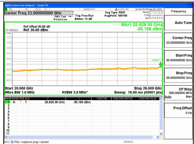
7A-12A-20G-26G / 20+10MHz / QPSK / High+Low CH / 1@99-1@0
