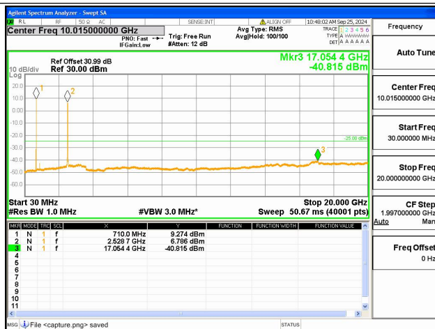
7A-12A-30M-20G / 20+10MHz / QPSK / Mid+High CH / 100@0-50@0
