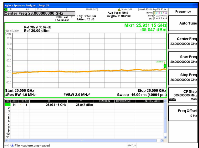
7A-12A-20G-26G / 20+10MHz / QPSK / Mid+Low CH / 1@0-1@49
