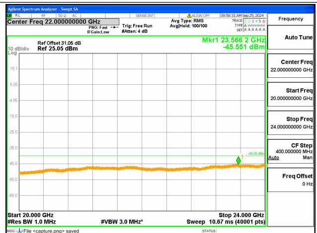
5A-30A-20G-24G / 10+10MHz / QPSK / Low+Low CH / 1@49-1@0
