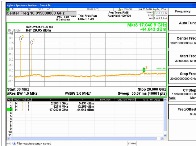
5A-30A-30M-20G / 10+10MHz / QPSK / Low+Low CH / 50@0-50@0
