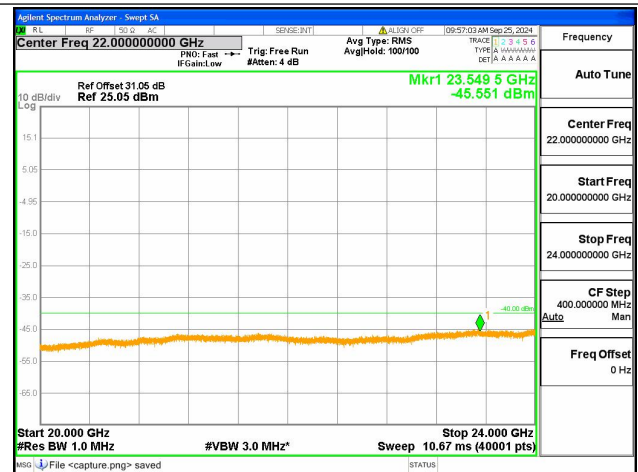
5A-30A-20G-24G / 10+10MHz / QPSK / Low+Mid CH / 1@0-1@49
