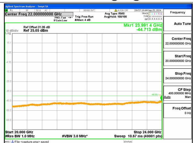
5A-30A-20G-24G / 10+10MHz / QPSK / Low+Mid CH / 1@49-1@0
