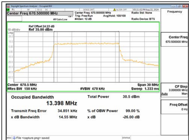
B71 / 15MHz / QPSK/ Low CH
