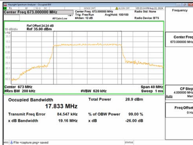
B71 / 20MHz / 64QAM/ Low CH
