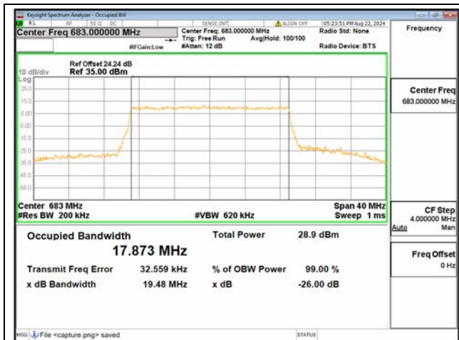
B71 / 20MHz / 64QAM/ Mid CH
