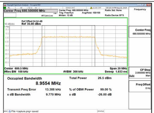
B71 / 10MHz / 256QAM/ Mid CH
