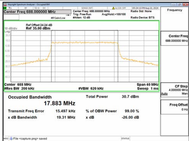
B71 / 20MHz / QPSK/ High CH
