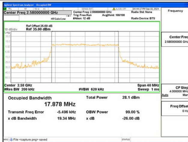
B38 / 20MHz / 64QAM/ Low CH
