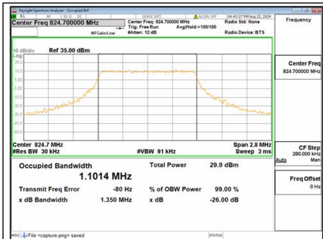
B26 Part22 / 1.4MHz / QPSK/ Low CH
