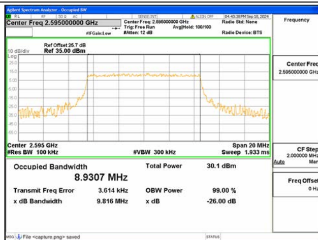
B38 / 10MHz / QPSK/ Mid CH
