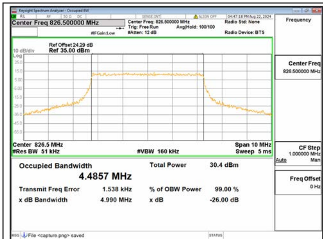
B26 Part22 / 5MHz / QPSK/ Low CH
