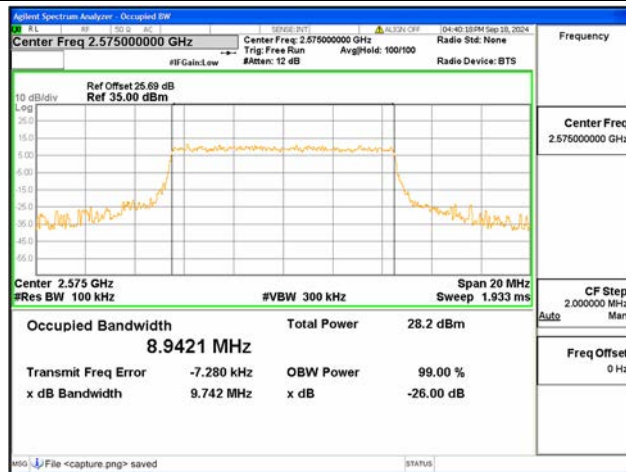
B38 / 10MHz / 64QAM/ Low CH
