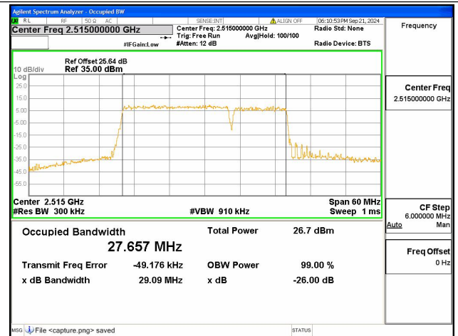
7C / 20+10MHz / 256QAM/ Low CH
