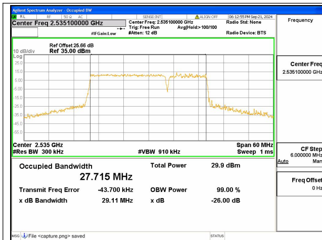
7C / 20+10MHz / QPSK/ Mid CH
