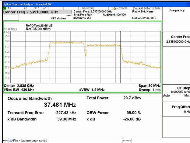
7C / 20+20MHz / QPSK/ Mid CH
