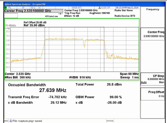
7C / 20+10MHz / 256QAM/ Mid CH
