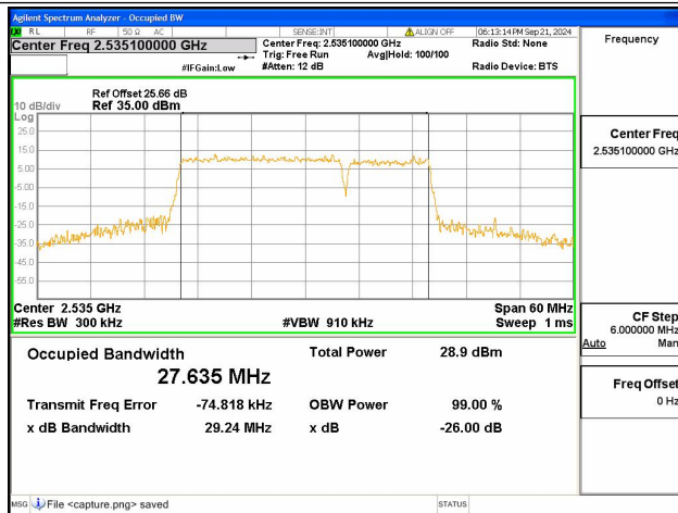
7C / 20+10MHz / 64QAM/ Mid CH
