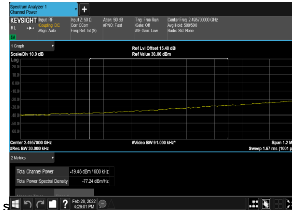
B2_N41(60M)_DFT-s- OFDM_QPSK_Edge_1RB_Left_Low_CH_chp_pas
