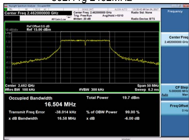
802.11g 2462MHz
