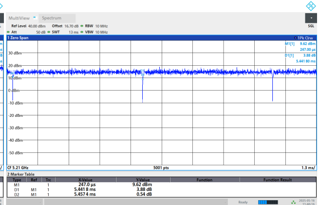
802.11ax(HE80)
