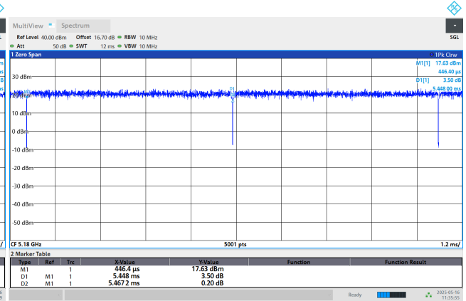
802.11ax(HE20)
