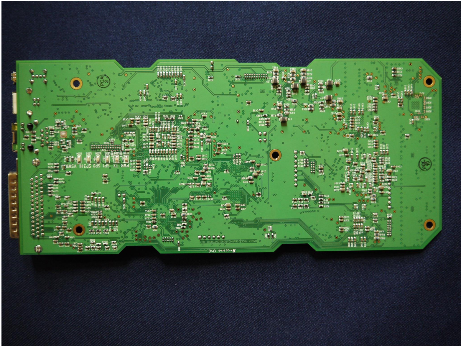
CMU PCB Bottom
