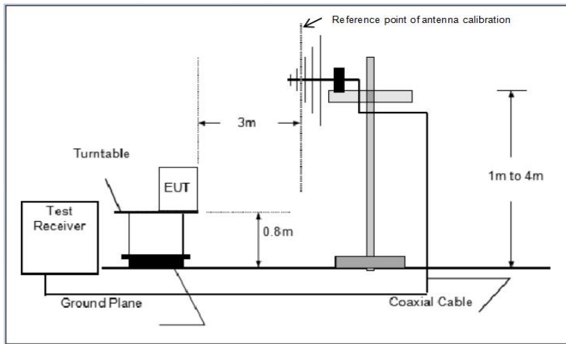
Below 1000MHz Test Setup
