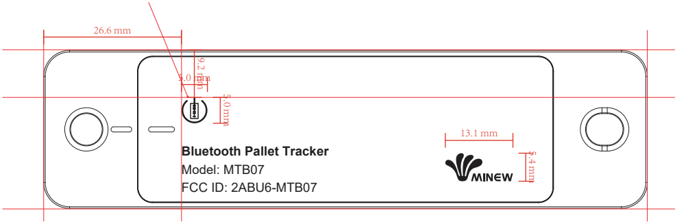
磁控开机元器件所在位置
