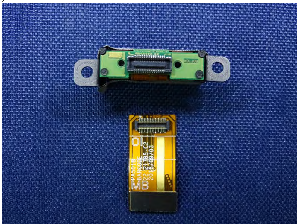
(88) EUT Photo
