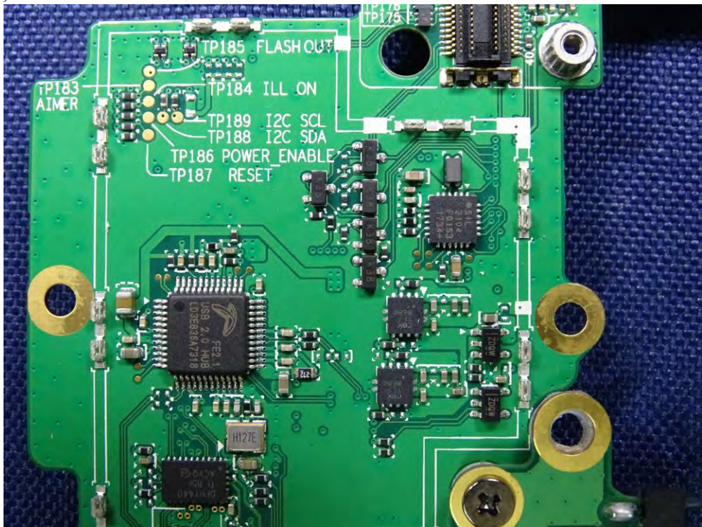
(58) EUT Photo
