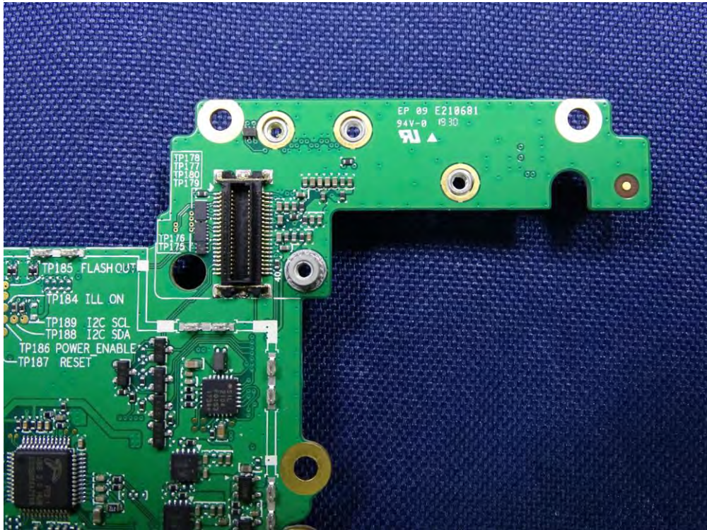
(57) EUT Photo
