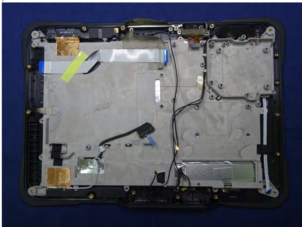
(74) EUT Photo
