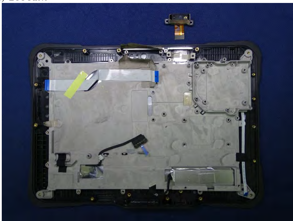
(86) EUT Photo
