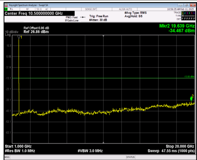
Band4-20MHz-QPSK-20300-1RB#0-Range2:1000~2 0000MHz
