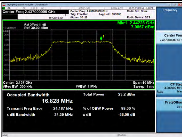
11G-Ant1-2437
