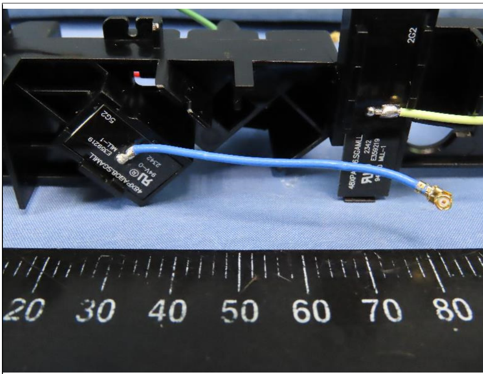
5G2 Antenna
