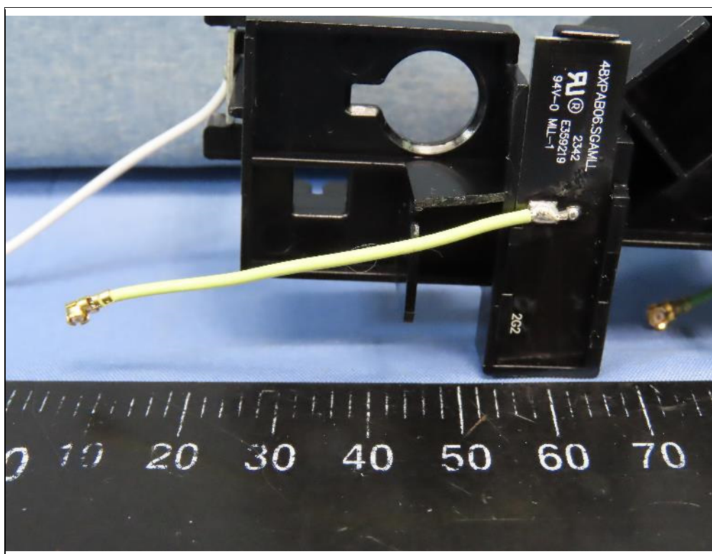
2G2 Antenna
