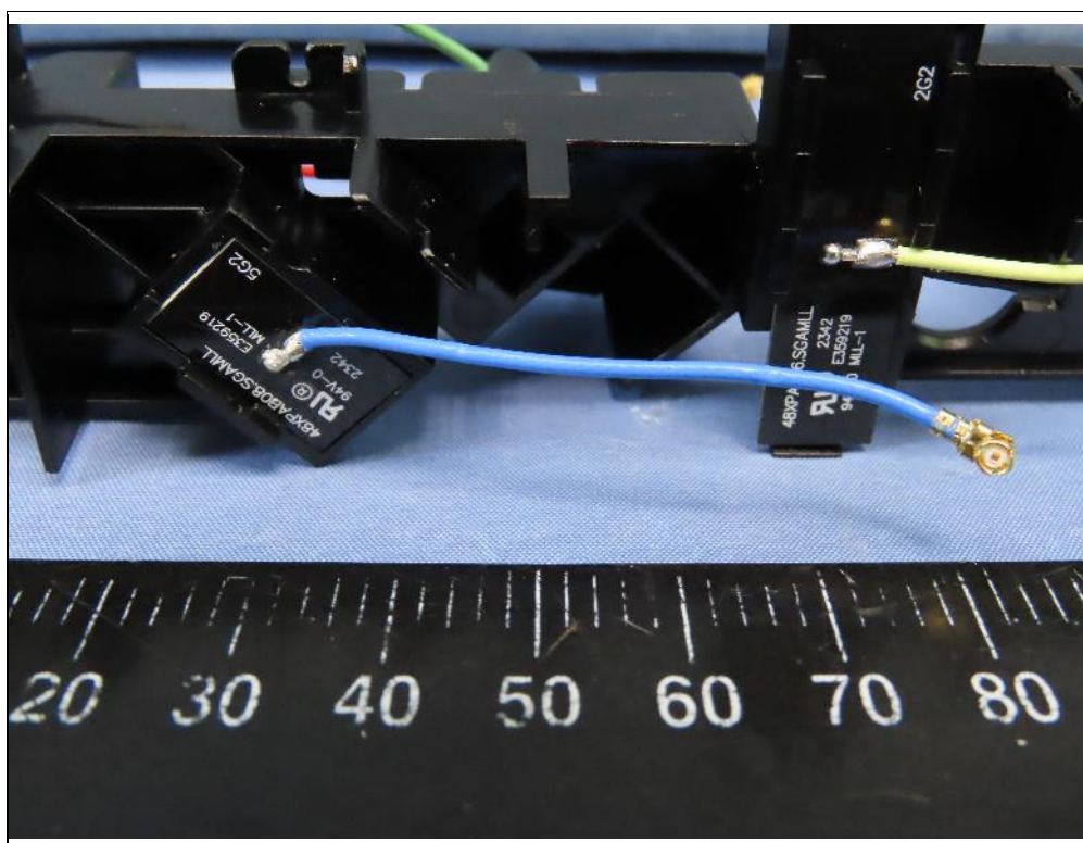
5G2 Antenna
