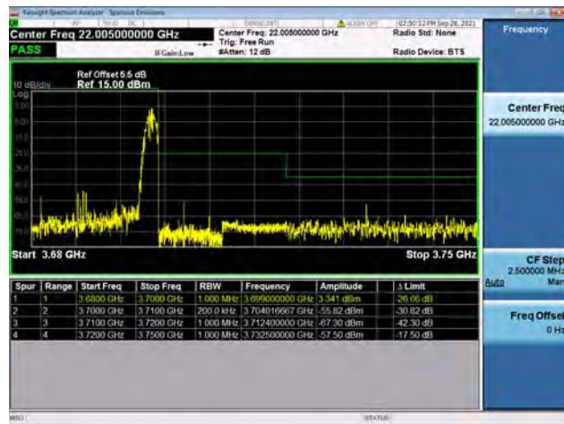
Band48 / 20MHz / High CH / QPSK / 1 RB
