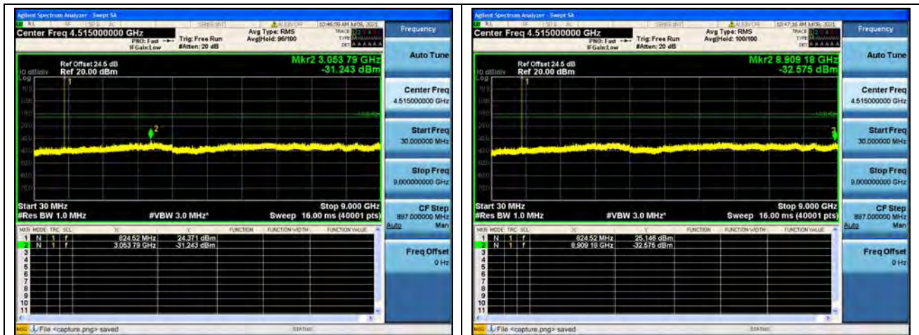
Band5 / 1.4MHz / Low CH / 64QAM
