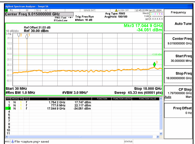
13A-66A / 10+20MHz / QPSK / Low+Mid CH / 1@0-1@99
