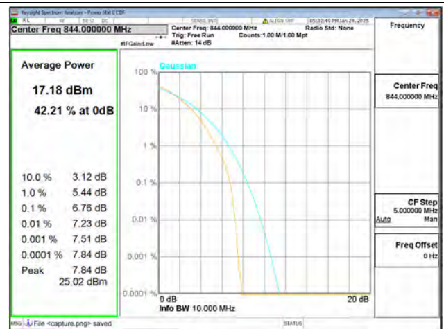
B5 / 10MHz / High CH / 64QAM
