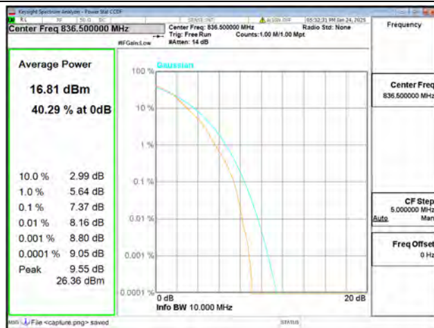
B5 / 10MHz / Mid CH / 64QAM
