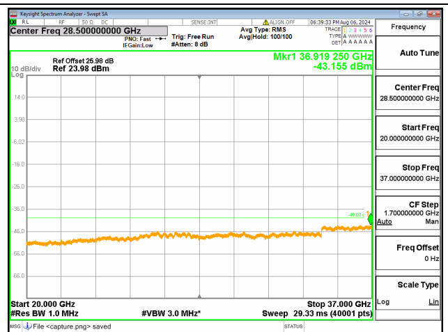
48C-20G-37G / 15+20MHz / QPSK / Mid CH / 1@0-1@99
