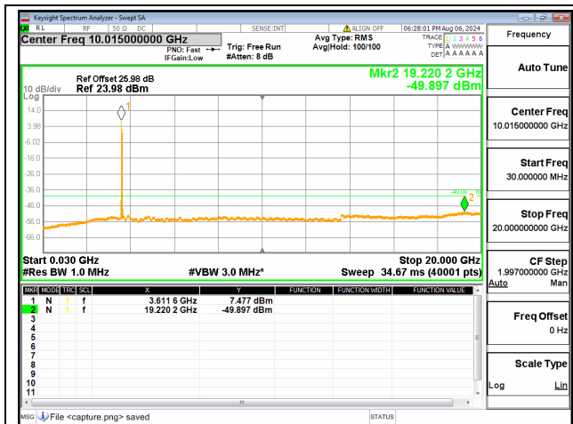
48C-30M-20G / 10+20MHz / QPSK / Mid CH / 1@0-1@99
