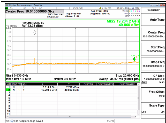
48C-30M-20G / 5+20MHz / QPSK / Mid CH / 1@0-1@99
