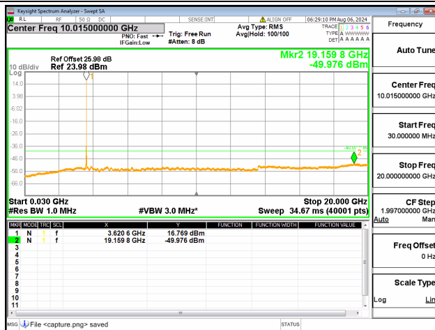
48C-30M-20G / 10+20MHz / QPSK / Mid CH / 1@49-1@0
