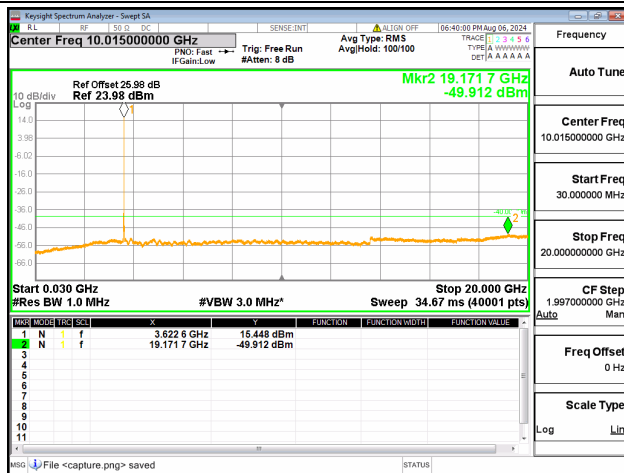
48C-30M-20G / 15+20MHz / QPSK / Mid CH / 1@74-1@0
