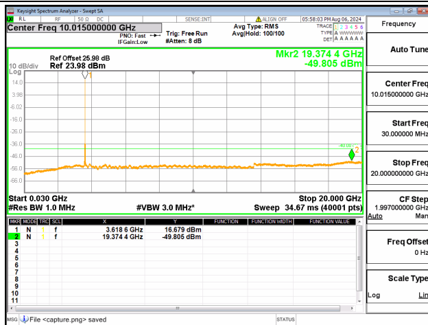
48C-30M-20G / 5+20MHz / QPSK / Mid CH / 1@24-1@0
