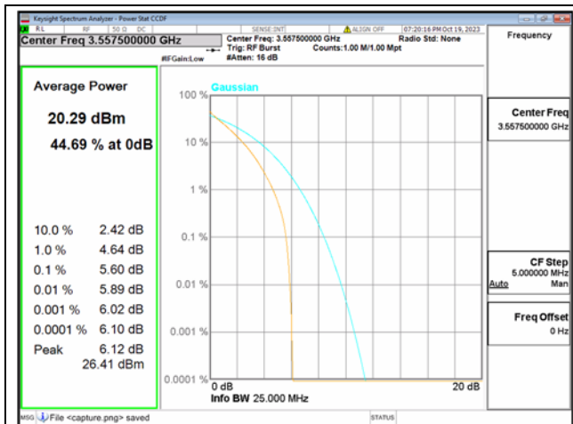
B48 / 15MHz / Low CH / QPSK
