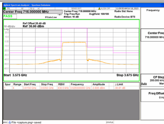
B48 / 20MHz / Mid CH / QPSK / FULL RB
