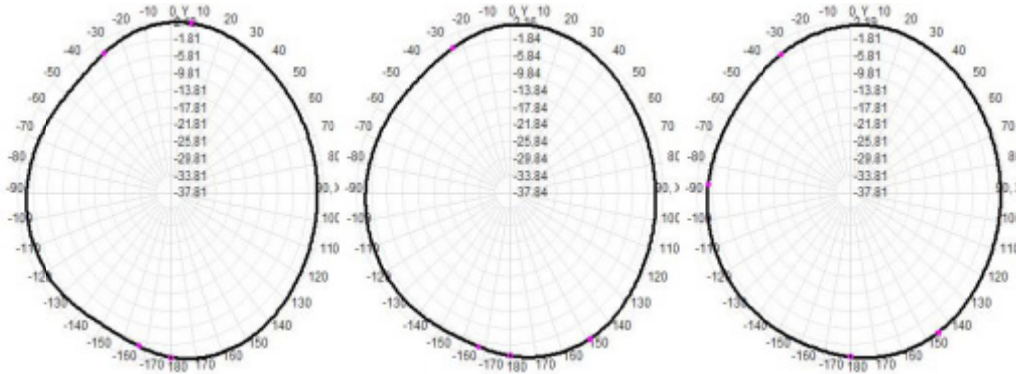
二：Antenna2D（2400MHz/2450MHz/2500MHz）
