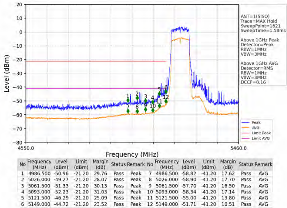
802.11ac(VHT80)_MCH_5210MHz_Ant1_NTNV
