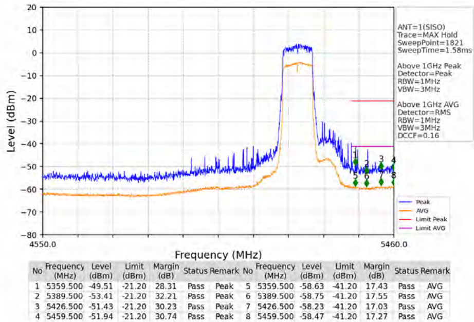
802.11ac(VHT80)_MCH_5210MHz_Ant1_NTNV
