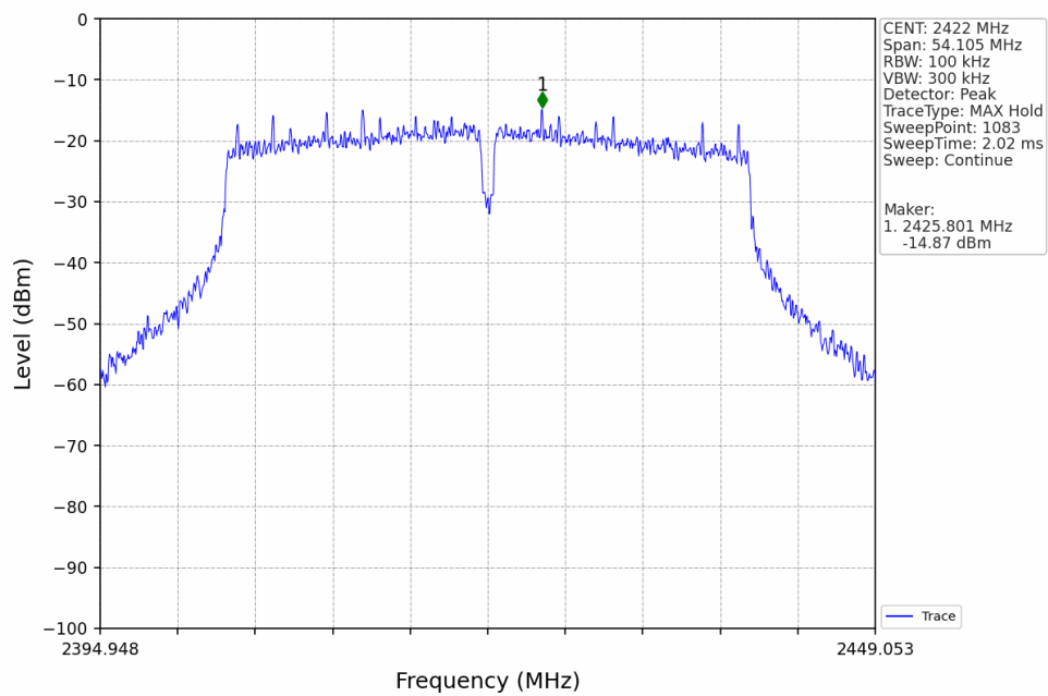
802.11n(HT40)_LCH_2422MHz_Ant1 (SISO)_NTNV
