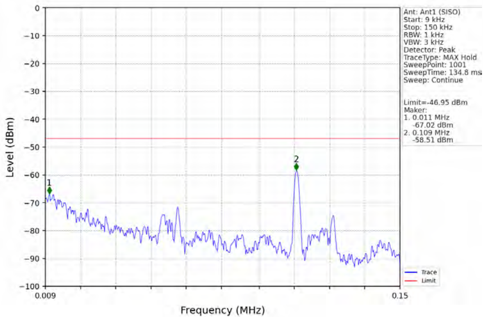
802.11n(HT20)_LCH_2412MHz_Ant1 (SISO)_NTNV
