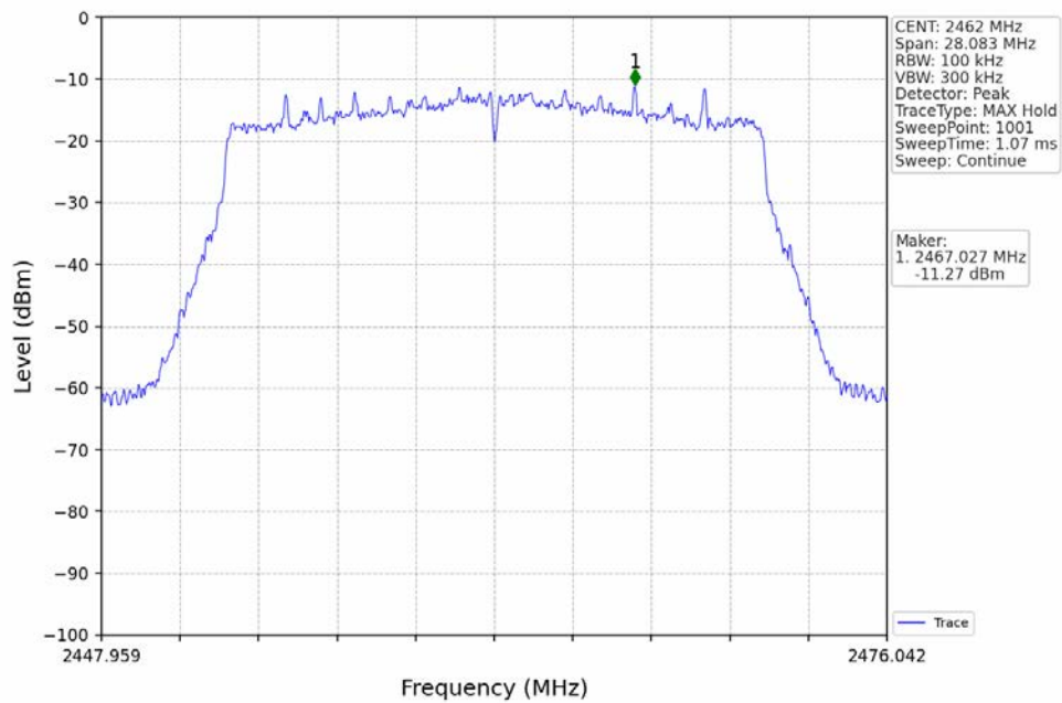
802.11ax(HEW20) HCH 2462MHz_RU242_Left_Ant2 (MIMO)_NTNV
