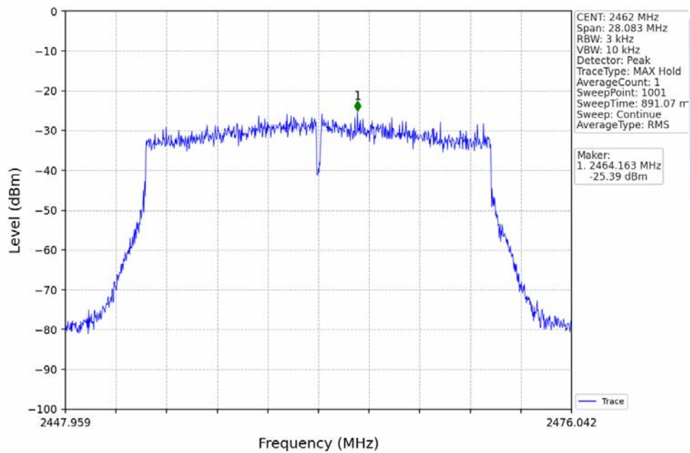
802.11ax(HEW20) HCH 2462MHz RU242 Left_Ant2 (MIMO) NTN
