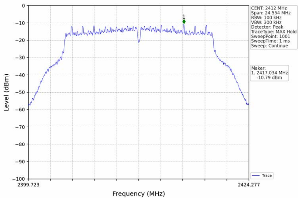
802.11g_LCH_2412MHz_Ant2 (SISO)_NTNV
