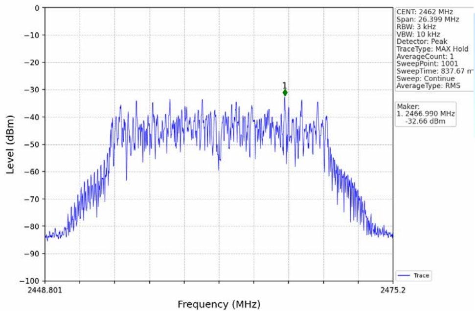
802.11n(HT20)_HCH_2462MHz_Ant2 (MIMO)_NTNV
