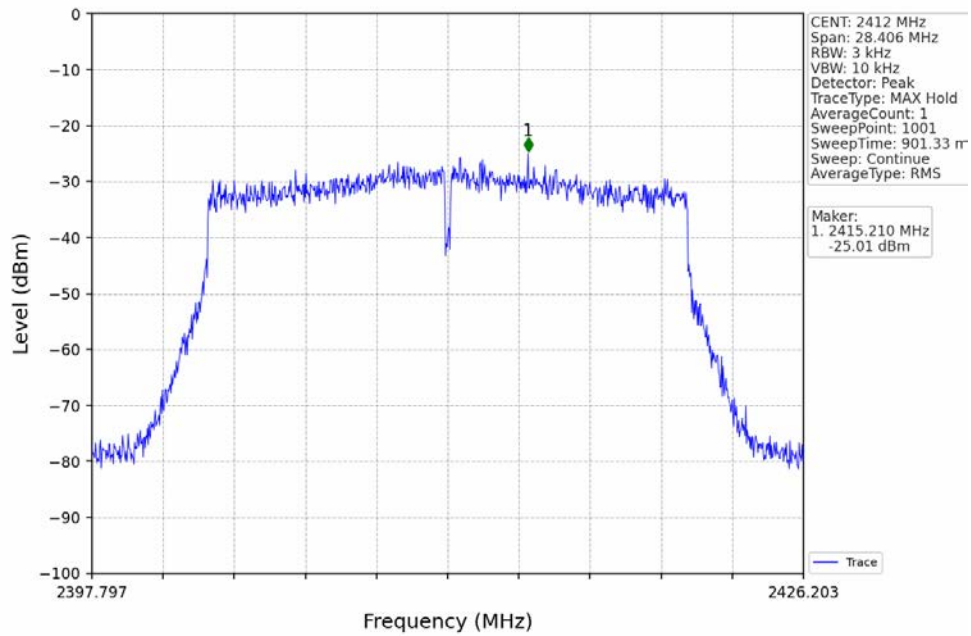
802.11ax(HEW20) LCH_2412MHz_RU242_Left_Ant2 (MIMO)_NTNV
