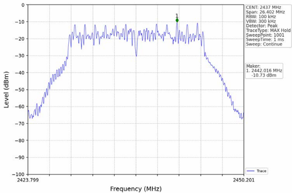
802.11n(HT20)_MCH_2437MHz_Ant2 (MIMO)_NTNV
