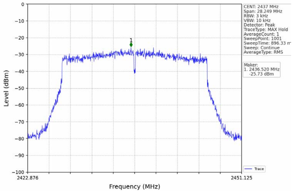
802.11ax(HEW20)_MCH_2437MHz_RU242_Left_Ant2 (MIMO)_NTNV
