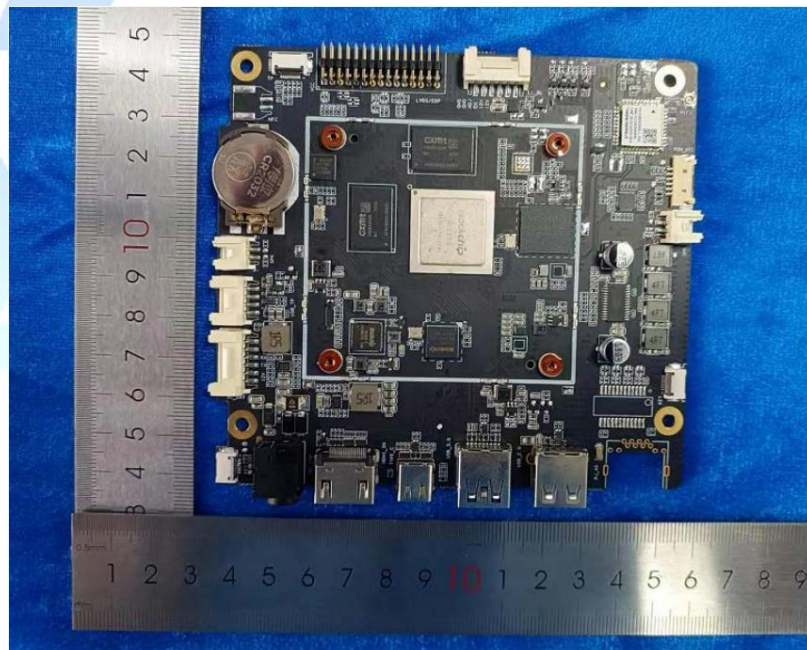
主板正面 (主板方案2) (适用于型号: SW2193T)
