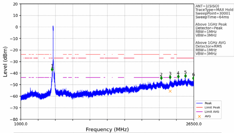
802.11ax(HEW80)_MCH_5775MHz_RU996_Left_Ant1_NTNV
