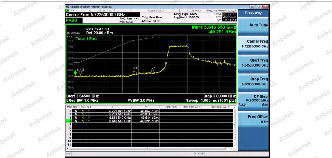
11AX80SISO-Ant1-5775-242Tone-RU61-PASS
