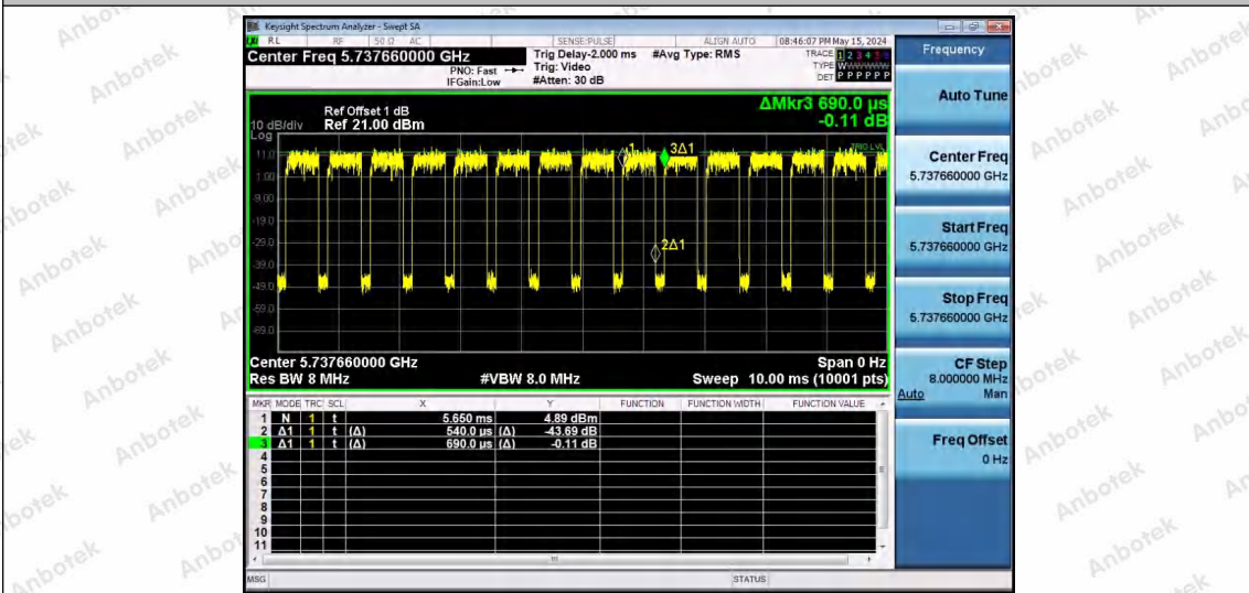
NTNV-11AX80SISO-Ant1-5775-52Tone-RU37
