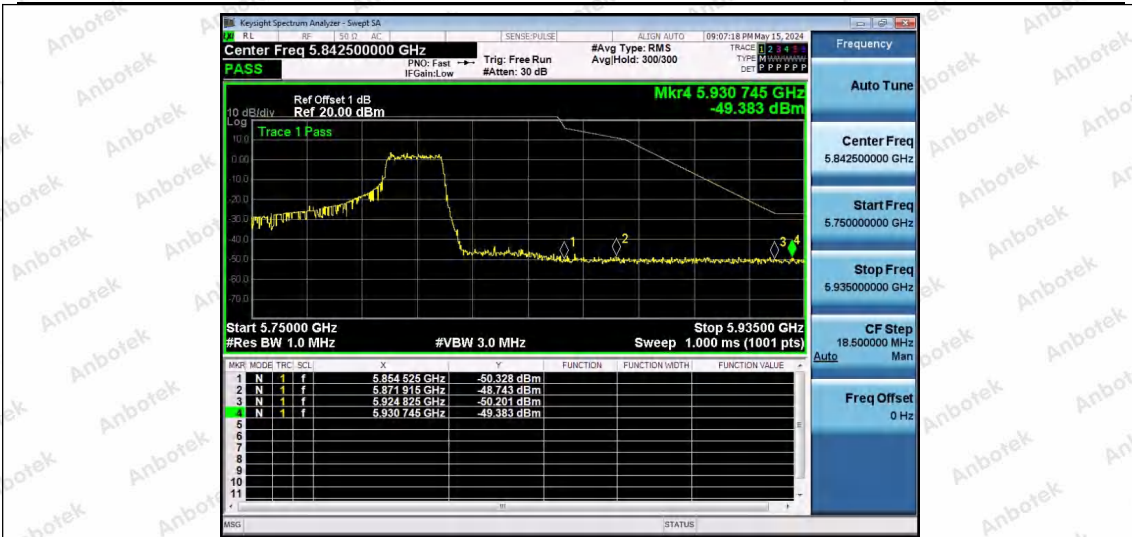
11AX80SISO-Ant1-5775-242Tone-RU64-PASS
