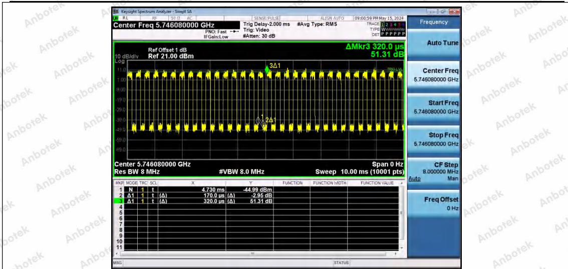
NTNV-11AX80SISO-Ant1-5775-242Tone-RU61
