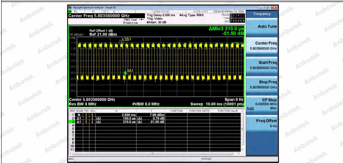
NTNV-11AX80SISO-Ant1-5775-242Tone-RU64
