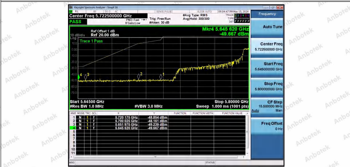
11AX80SISO-Ant1-5775-242Tone-RU64-PASS
