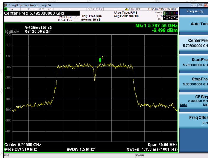
11AC40SISO_Ant2_5795
