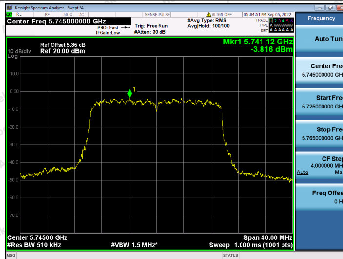
11AX20SISO_Ant2_5745
