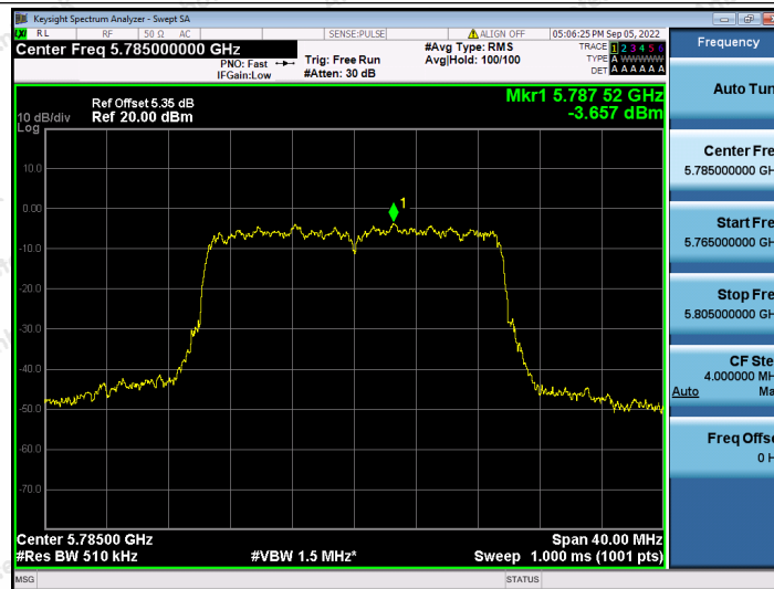
11AX20SISO_Ant2_5785
