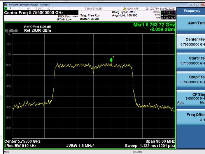
11AX40SISO_Ant2_5755
