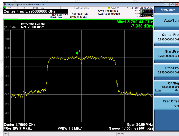
11AX40SISO_Ant2_5795
