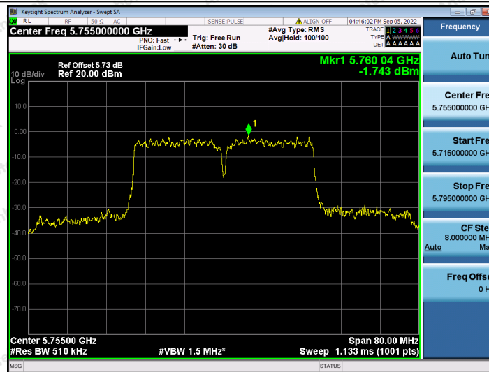
11N40SISO_Ant2_5755
