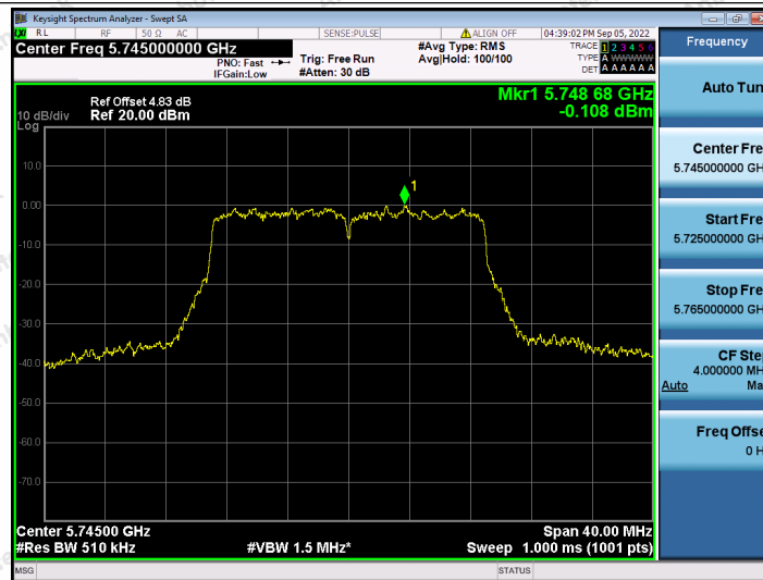
11N20SISO_Ant2_5745
