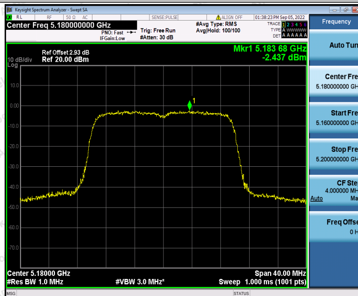
11AX20SISO_Ant2_5180
