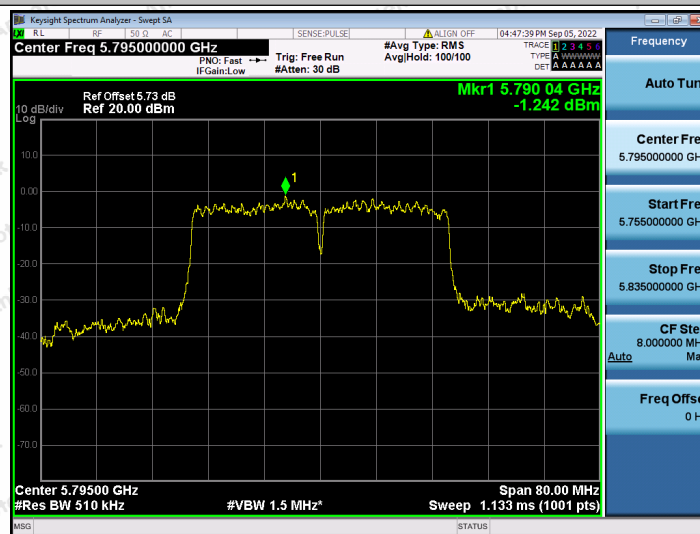
11N40SISO_Ant2_5795
