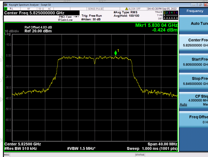
11N20SISO_Ant2_5825
