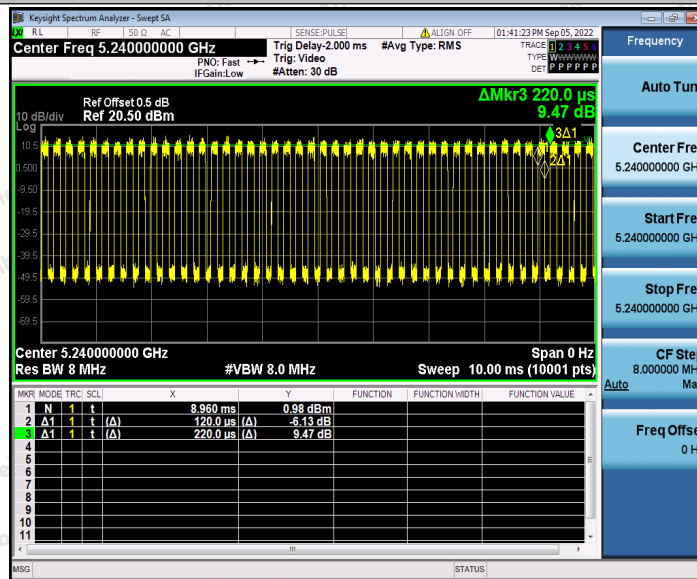
11AX20SISO_Ant2_5240
