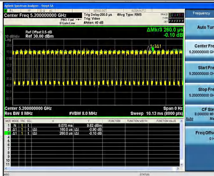
11N20SISO_Ant2_5200
