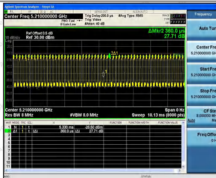
11AX80SISO_Ant2_5210
