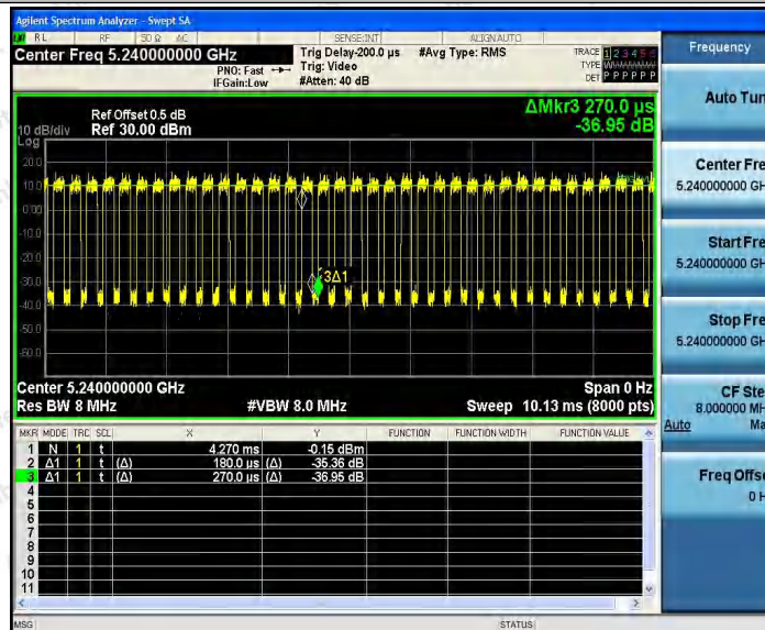
11A_Ant2_5240
