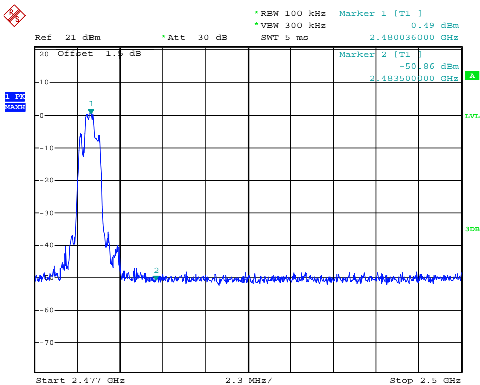
(Plot 4.5.2.3 B: Hopping Mode @ \pi/4 DQPSK)
