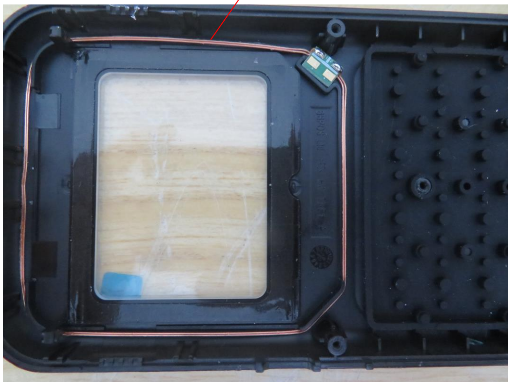
NFC Antenna
