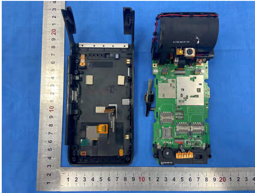
NFC antenna
