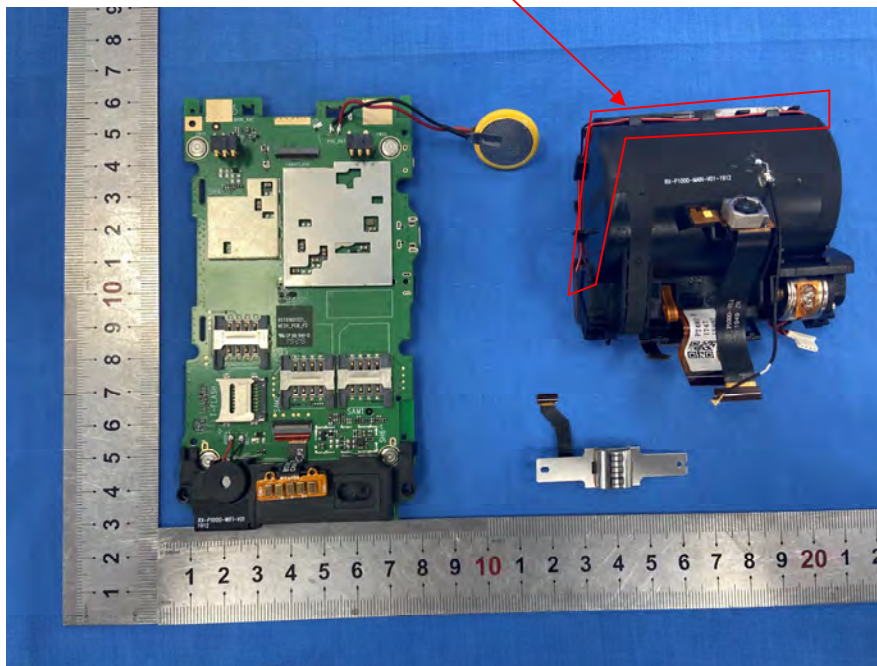
NFC antenna
