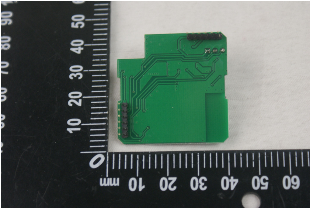
THE MIAN BOARD 2 (Rear)
