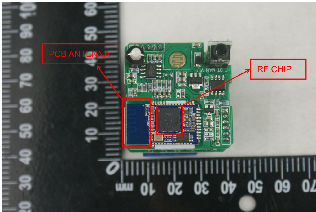
THE MIAN BOARD
