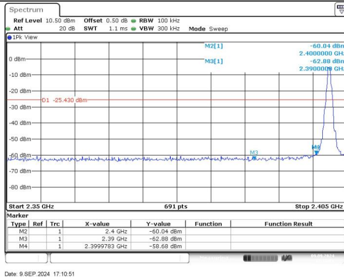
DH5_Ant1_Low_2402
