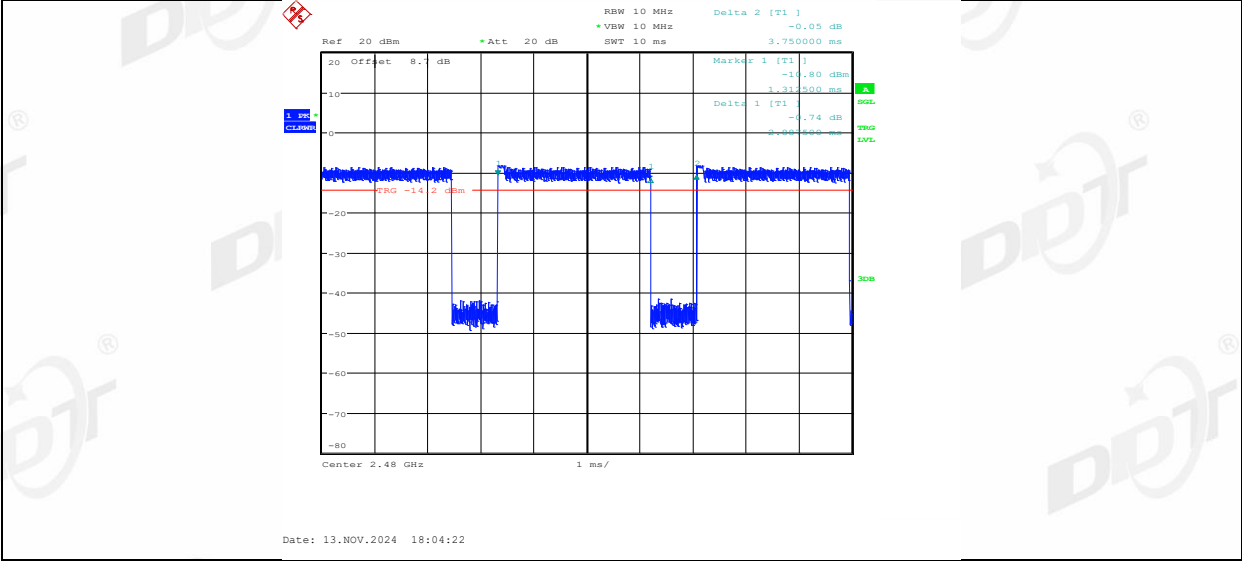
NTVN_3DH5_Ant1_2480
